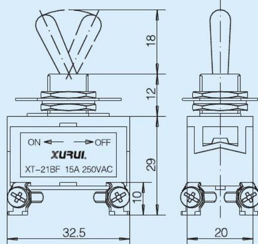
• 双极单向自动复位型 DPST REINICIO AUTOMATICO (ON)-OFF XT-21BF
