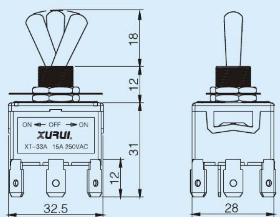
• 三极双投中间停型 TPDT ON-OFF-ON XT-33A
