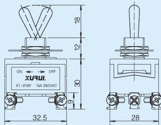
• 三极单向自动复位型 TPST REINICIO AUTOMATICO (ON)-OFF XT-31BF
